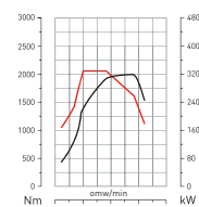
DTI 11 - 430 PK
