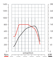
DTI 5 - 210 PK
